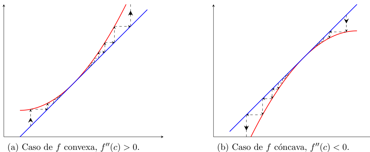
Figura 1.4: Idea intuitiva de la demostración.
