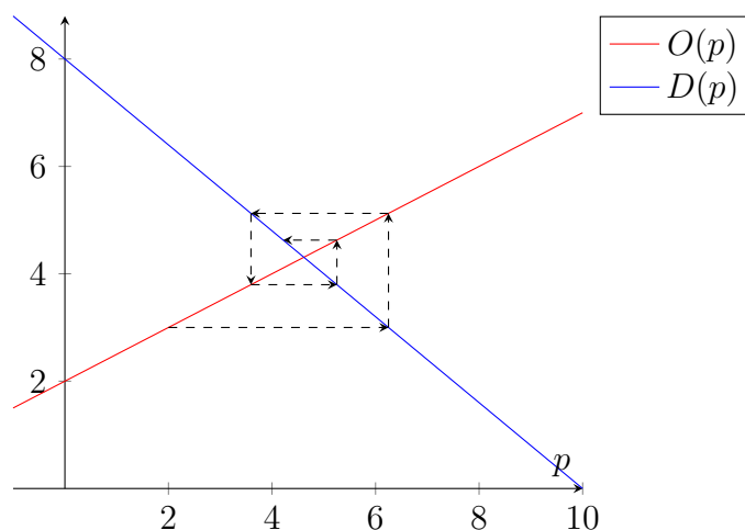
Figura 1.1: Representación del modelo de la Telaraña.
